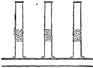
चित्र १०४—सेरापिस का मंदिर
